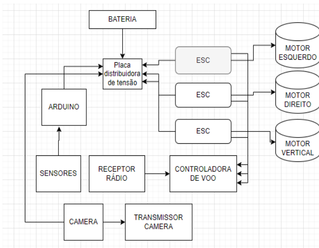
Figura 4: Diagrama de Blocos.
