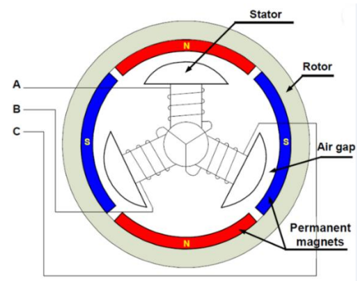
Figura 5: Vista em Corte de Um Motor BLDC.
