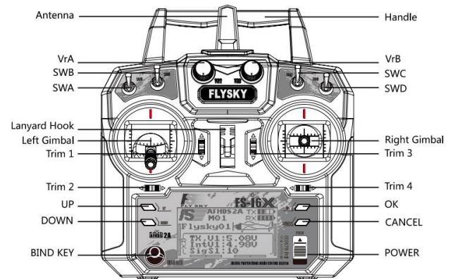
Figura 6: visão geral do rádio FlySky FS-i6X.
