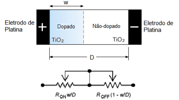
Figura 2: Variáveis de estado de um memristor e representação de um memristor como uma associação em série de resistores (Adaptado de [10]).
