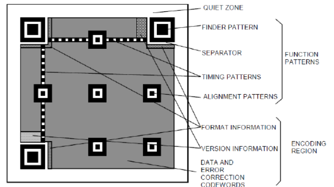
Figura 1: Regiões de um QR Code, ilustrado em símbolo da Versão 7 [7].
