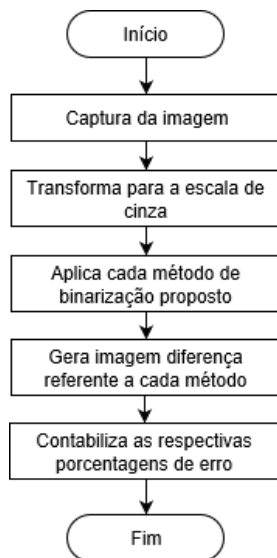
Figura 3: Fluxograma do procedimento realizado sobre cada imagem.
