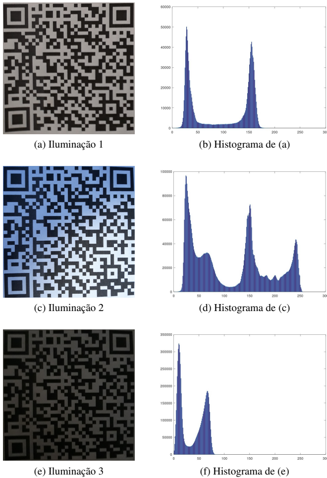
Figura 2: Exemplos de imagens de um mesmo QR Code nos três diferentes padrões de iluminação e seus respectivos histogramas.
