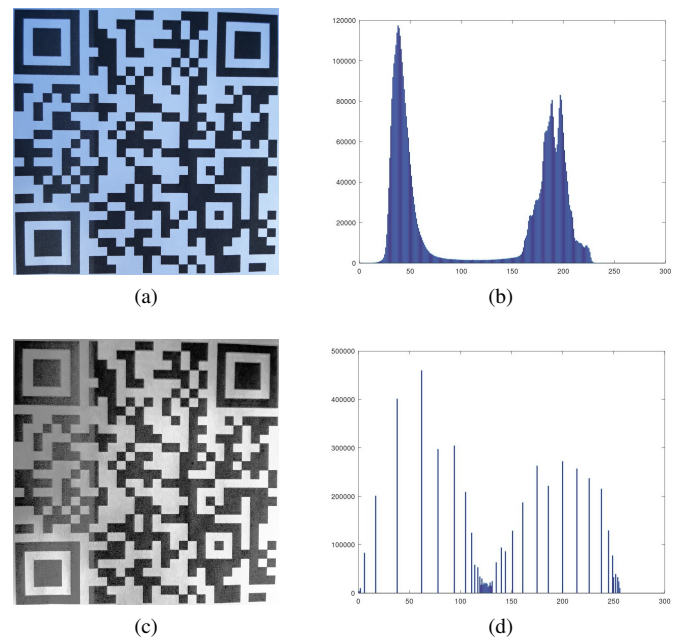
Figura 6: (a) QR Code 1 submetido ao padrão de Iluminação 2, (b) histograma de (a), (c) imagem resultante da equalização de histograma e (d) histograma de (c).
